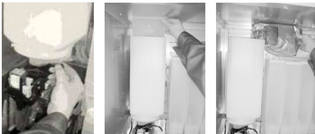
Рисунок 14 - Заполнение контейнера для кофе
