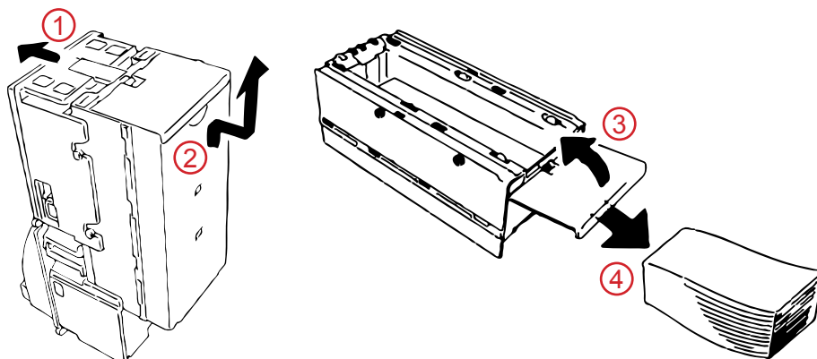
Рисунок 45 - Снятие и опустошение стекера
